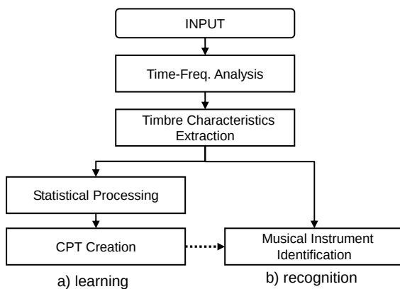
図 2 楽器同定処理部の詳細
