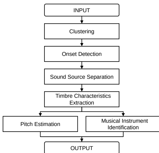
図1 自動採譜システムの構成
